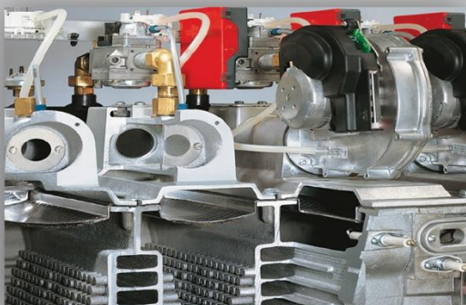
نمایی از پره های دیگ و ادوات کنترلی
